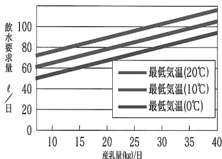
図1 産乳量、気温と飲水要求量の関係 (NRC2001年版より作成)
