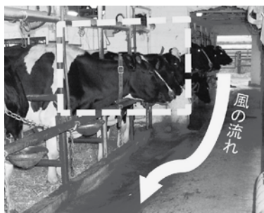
写真4 風の流れをさえぎる壁（黄色の点線部）は、建物の強度を保てる範囲でできるだけ開放する
