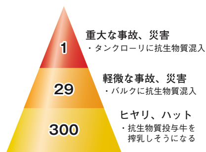
図1 ハイネリッヒの法則
