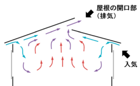
図1 フリーストール牛舎の換気構造
